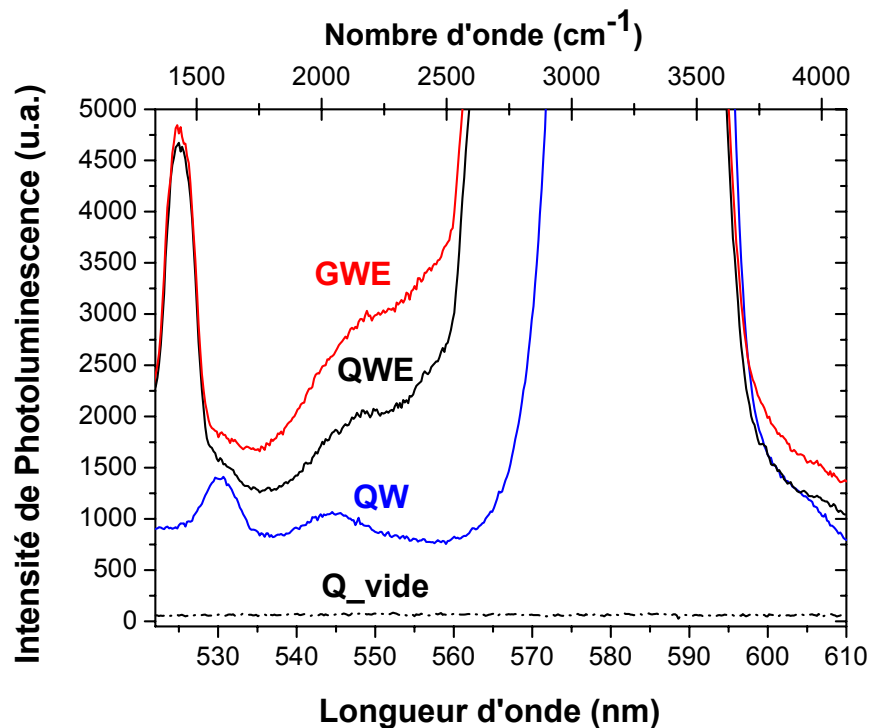
Figure II.5-6 : Spectres de photoluminescence (excitée à 488\text{ nm} ) d'une solution hydroalcoolique contenue dans les tubes en silice fondue (QWE), en verre sodocalcique de type III (GWE) et aussi de l'eau Seromed contenue dans des tubes en silice fondue (QW) ainsi que d'une cuve en silice fondue vide (Q). L'échelle supérieure des abscisses correspond au nombre d'onde associé à l'effet Raman (donc avec déduction de la longueur d'onde d'excitation).
