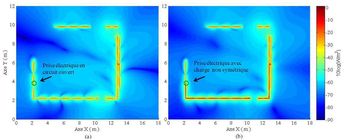
Figure 3.32 Rayonnement sans (a) et avec (b) une charge non symétrique connectée à une prise électrique
