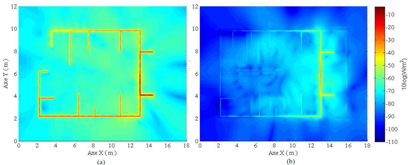
Figure 3.34 Densité de puissance du rayonnement (du CPL) dans une structure de maison type
